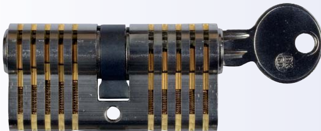
Modell "Starter" zylindrische Stifte im Kern und Gehäuse
